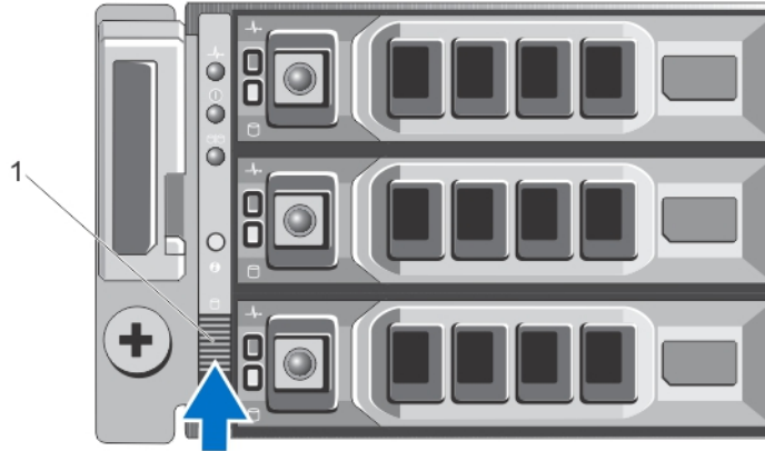
図 1. PowerVault MD1200 ストレージエンクロージャ設定スイッチの設定
